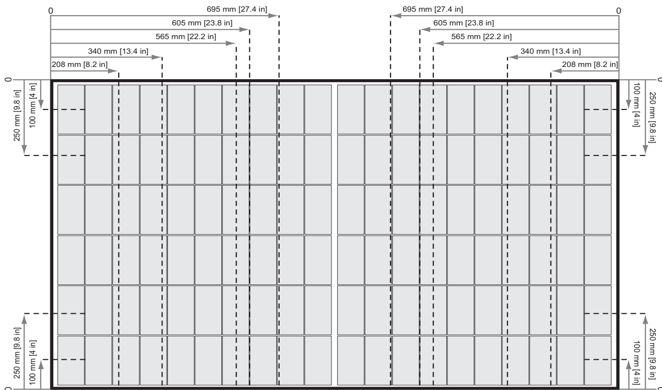
Rys. 3: Mocowanie paneli REC Alpha Series z szynami równoległymi do krótkiego boku panelu
