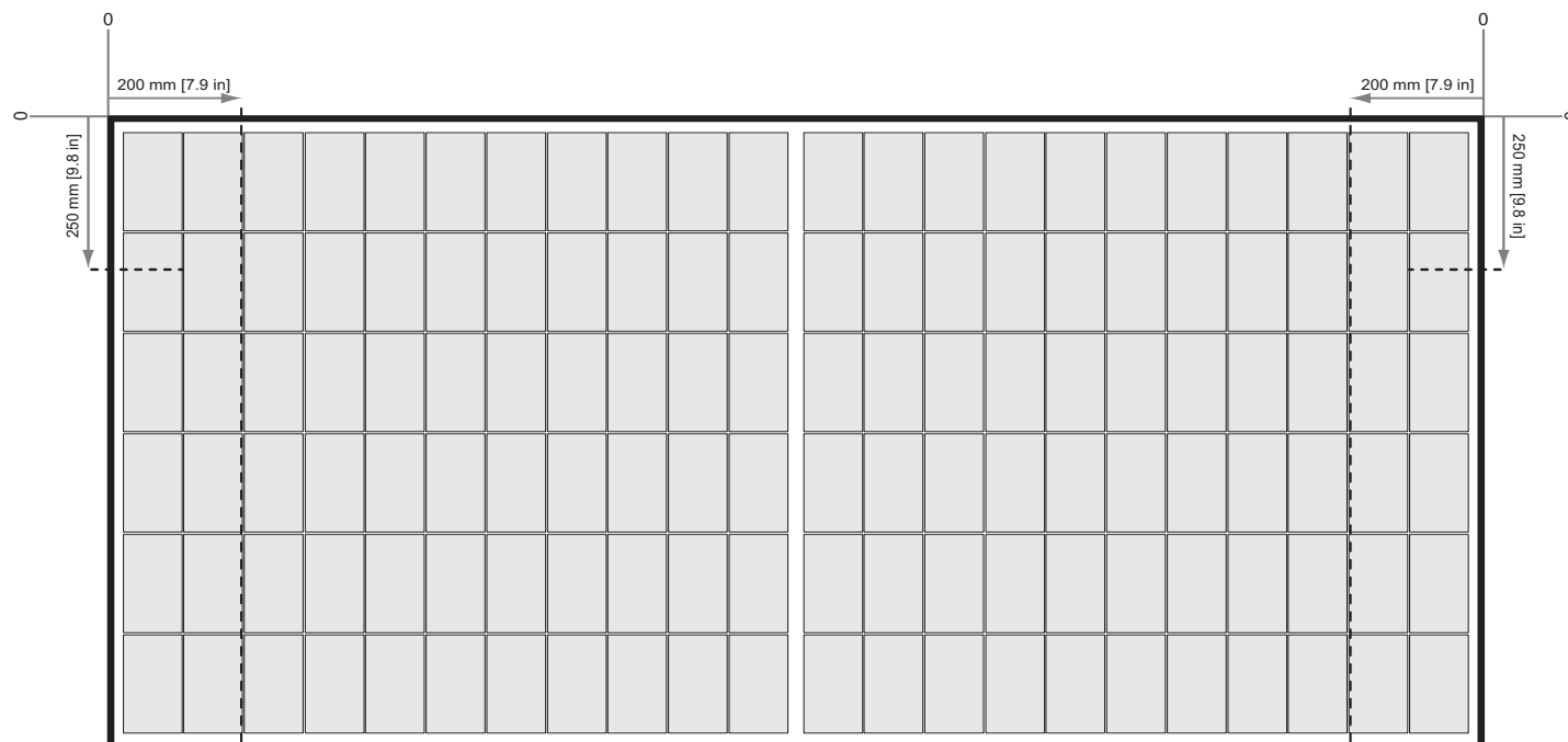
Rys. 10: Mocowanie paneli REC Alpha 72 Series z krótkimi szynami
