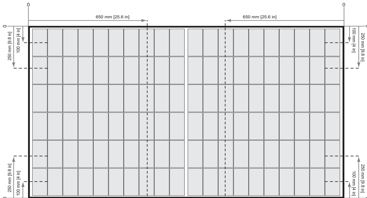
Rys. 4: Mocowanie paneli REC Alpha Series z szynami równoległymi do długiego boku panelu
