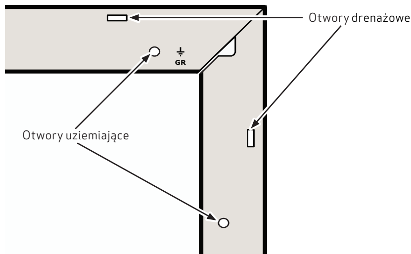
Rys. 15: Otwory drenażowe i uziemiające
