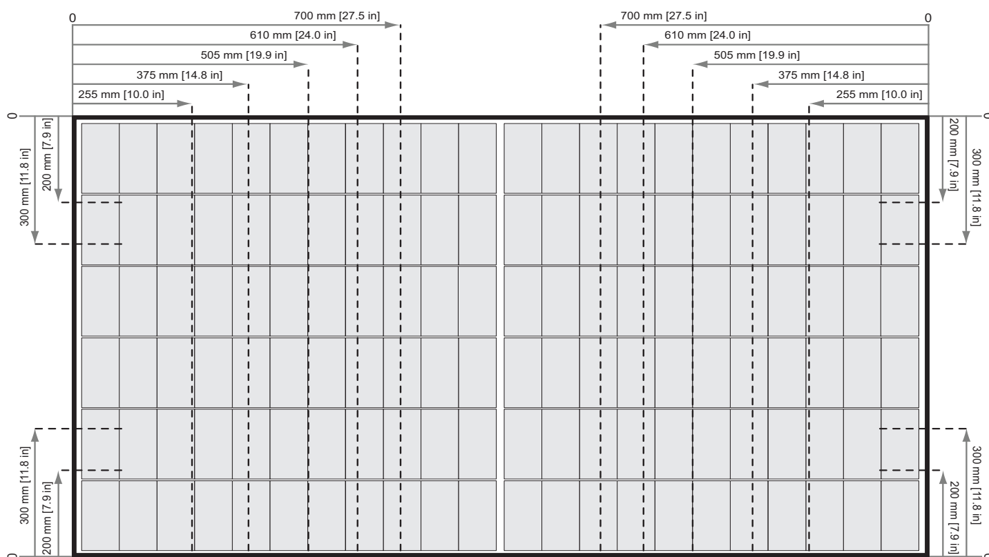
Rys. 6: Mocowanie paneli REC Alpha Pure Series z szynami równoległymi do krótkiego boku panelu
