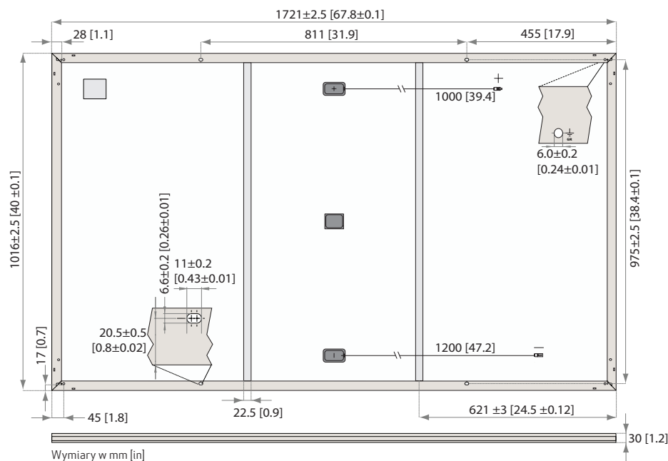
Rys. 18: Wymiary panelu: REC Alpha Series
