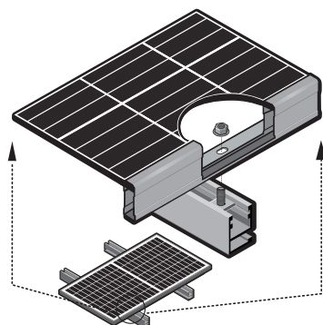
Rys. 14: Przykład instalacji otworu montażowego
