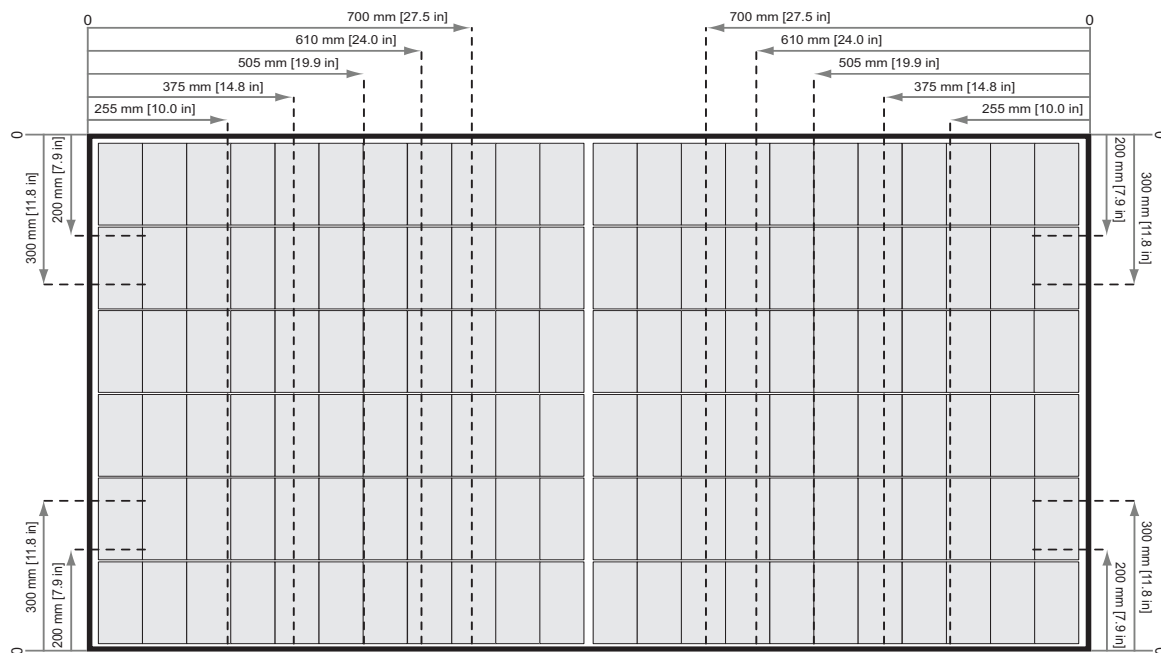
Rys. 8: Mocowanie paneli REC Alpha Pure Series z krótkimi szynami
