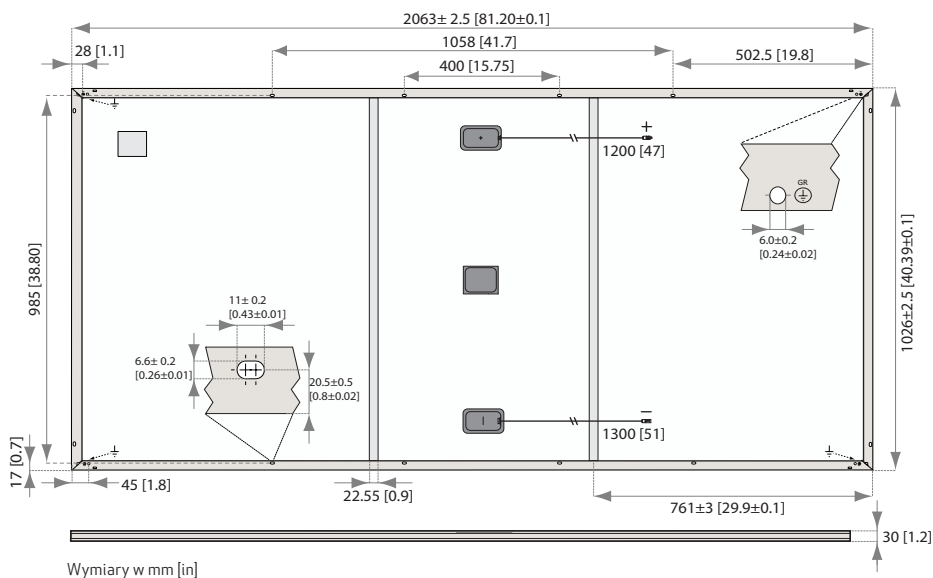
Wymiary w mm [in]
