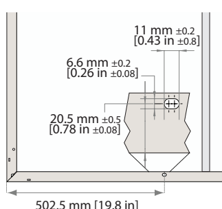
Rys. 12: Otwory montażowe: REC Alpha 72 Series
