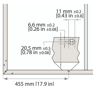
Rys. 11: Otwory montażowe: REC Alpha Series
