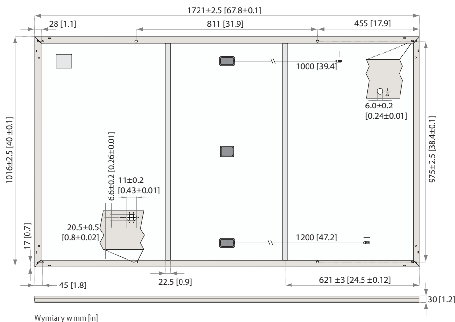
Rys. 19: Wymiary panelu: REC Alpha Black Series
