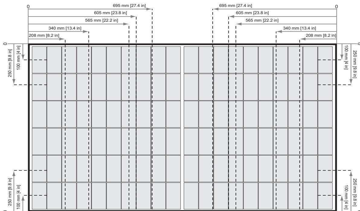
Rys. 5: Mocowanie paneli REC Alpha Series z krótkimi szynami
