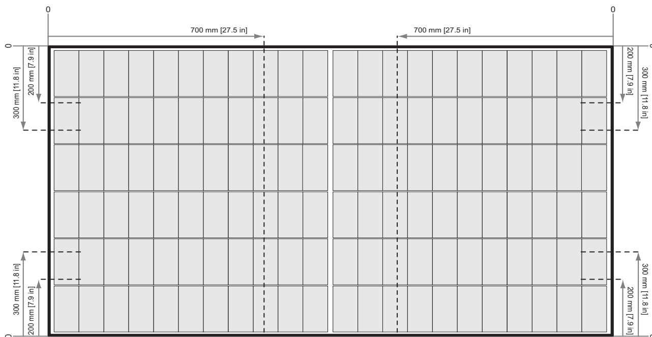
Rys. 7: Mocowanie paneli REC Alpha Pure Series z szynami równoległymi do długiego boku panelu
