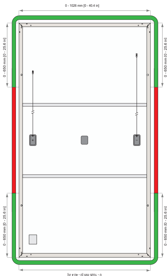
Rys. 23: Obszary instalacji urządzeń MLPE dla paneli REC Alpha 72 Series
