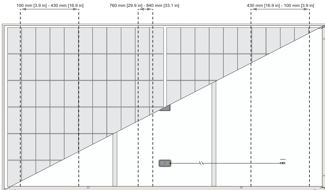
Rys. 24: Sześciopunktowe strefy mocowania
