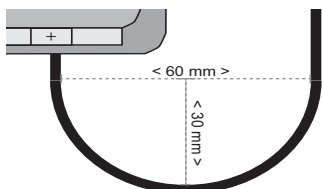
Rys. 16: Minimalny promień zagięcia kabla
