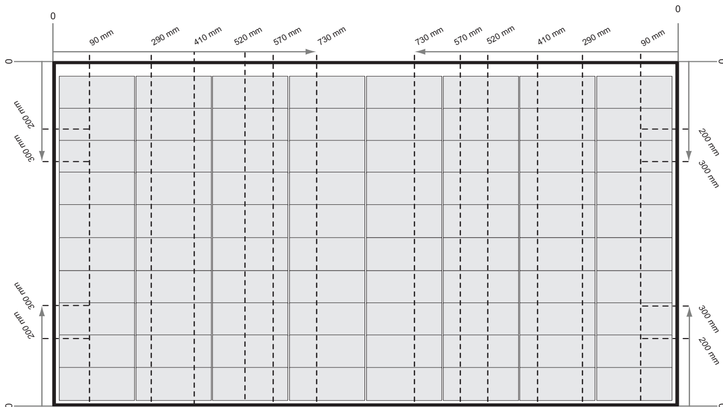
Abb. 6: Befestigung von Solarmodulen der REC Alpha Pure-R-Serie auf Schienen parallel zur kurzen Seite des Moduls
