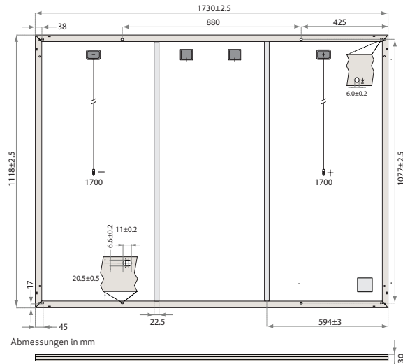
Abb. 18: Abmessungen: REC Alpha Pure-R-Serie
