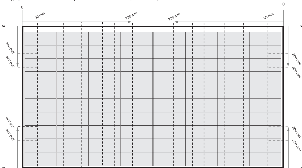
Abb. 7: Befestigung von Solarmodulen der REC Alpha Pure-R-Serie auf Schienen parallel zur langen Seite des Moduls
