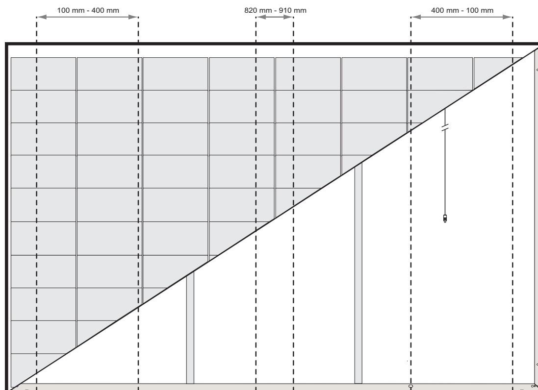
Abb. 13: Klemmzonen für Sechs-Punkt-Montage: REC Alpha Pure-R-Serie
