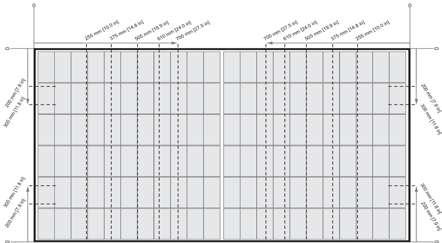
Abb. 3: Befestigung von Solarmodulen der REC Alpha Pure-Serie auf Schienen parallel zur kurzen Seite des Moduls
