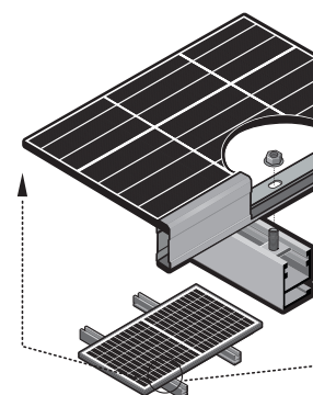
Abb. 11: Beispiel: Montage mit Hilfe der Montagelöcher
