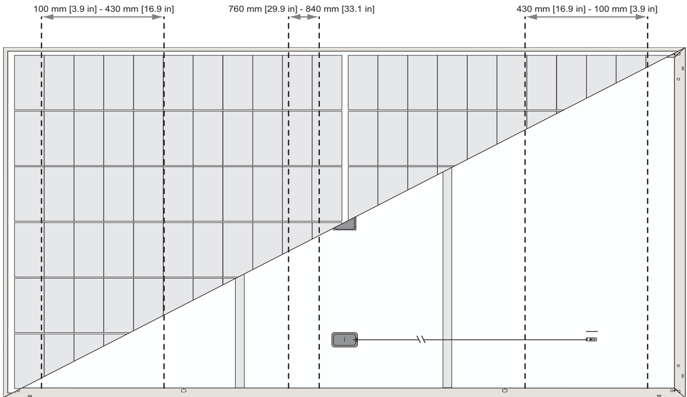
Abb. 12: Klemmzonen für Sechs-Punkt-Montage: REC Alpha Pure-Serie
