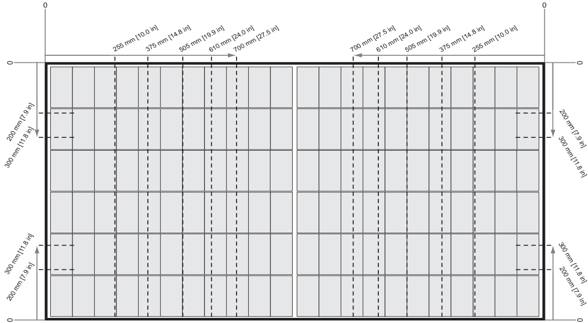
Abb. 5: Befestigung von Solarmodulen der REC Alpha Pure-Serie mit Kurzschienen
