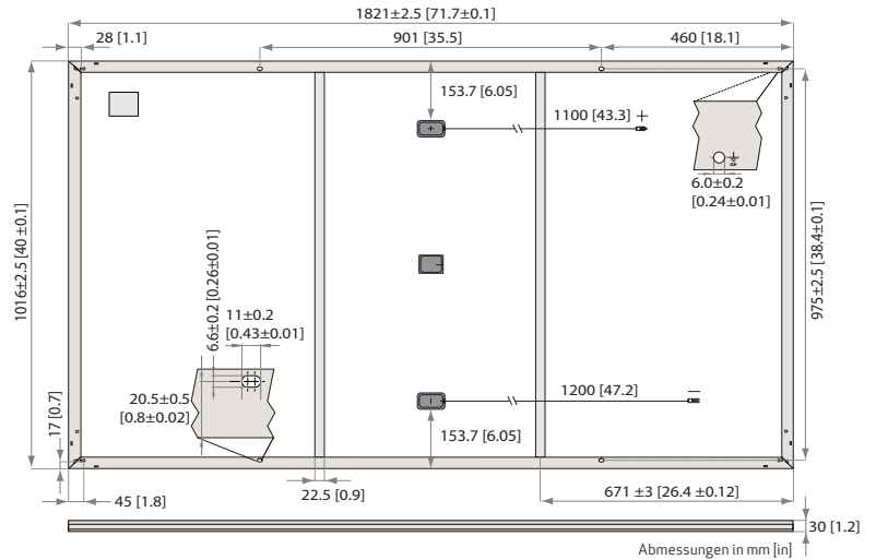
Abb. 17: Abmessungen: REC Alpha Pure-Serie
