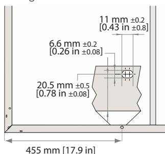
Abb. 9: Montagelöcher
