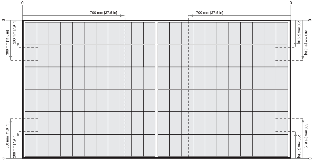
Abb. 4: Befestigung von Solarmodulen der REC Alpha Pure-Serie auf Schienen parallel zur langen Seite des Moduls
