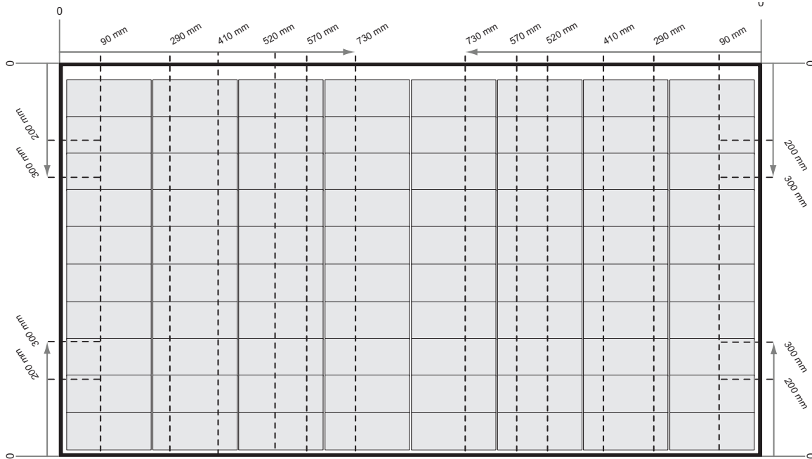
Abb. 8: Befestigung von Solarmodulen der REC Alpha Pure-R-Serie mit Kurzschienen
