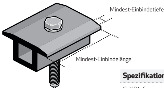
Abb. 1: Klemmenspezifikation
