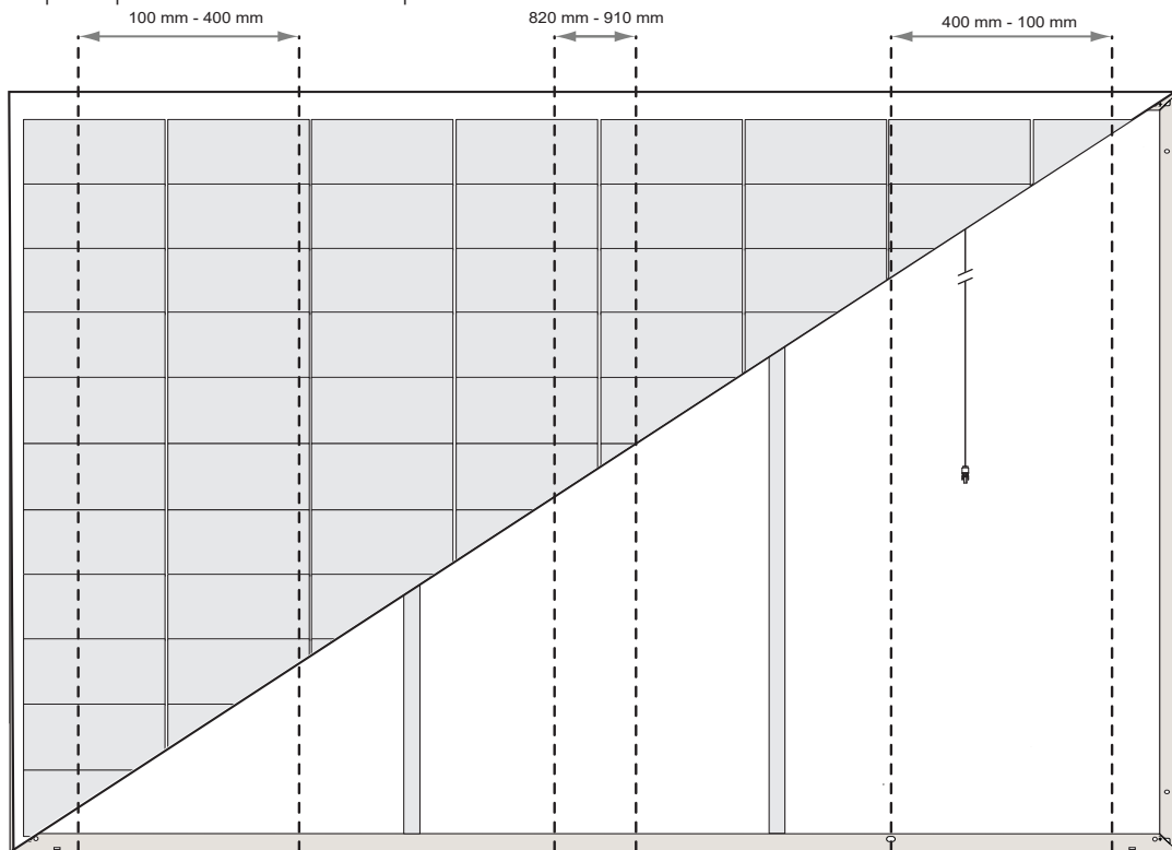
Afb. 5-4 Zespuntsopbouw klembereiken: REC Alpha Pure-RX serie
