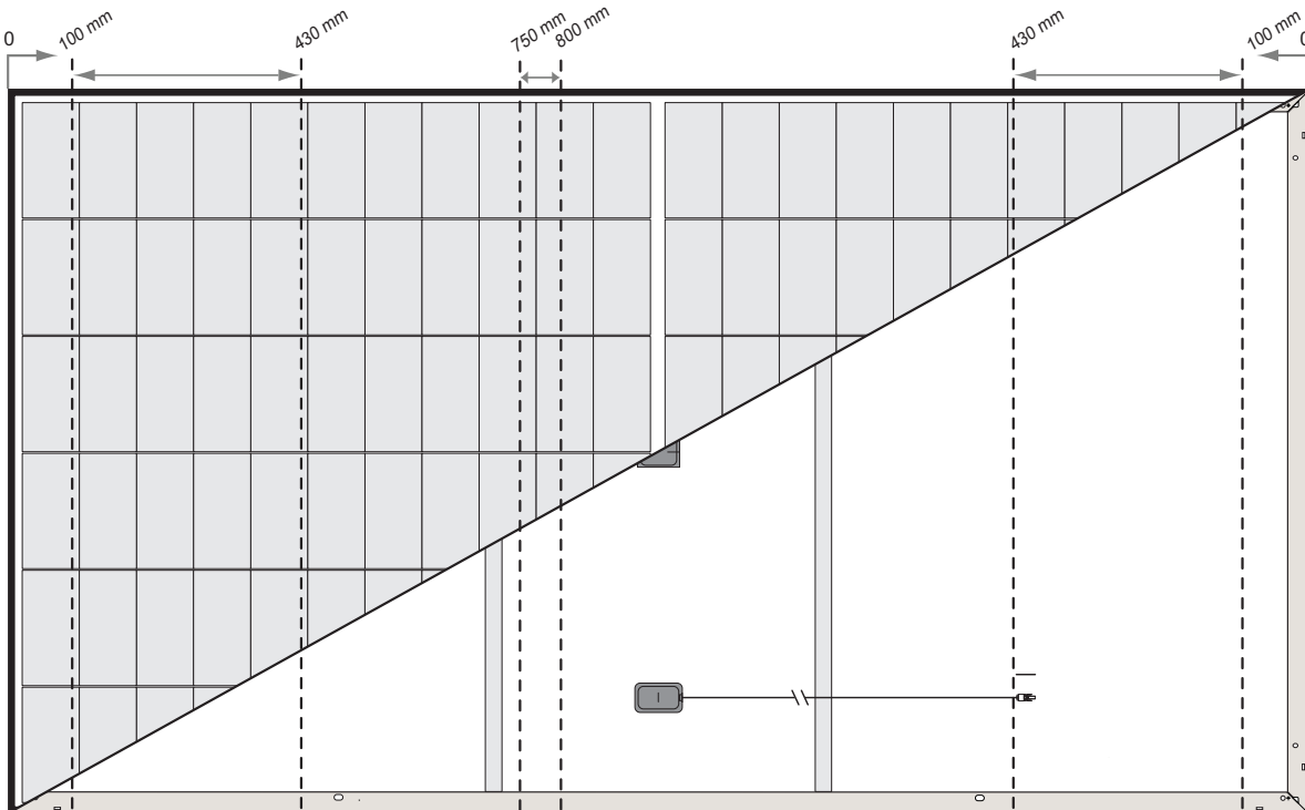
Afb. 3-4 Zespuntsopbouw klembereiken: REC Alpha Pure 2 serie
