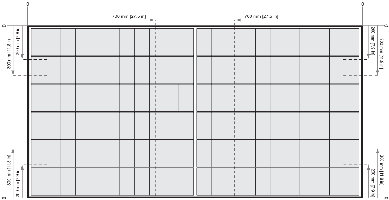
Afb. 2-2 Klemmen van REC Alpha Pure serie panelen met Rails parallel aan de lange zijde van het paneel
