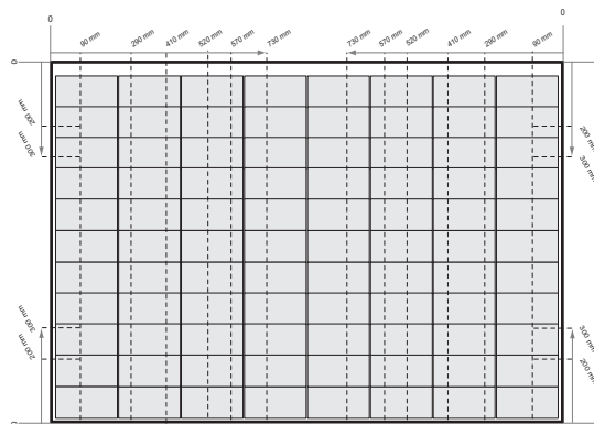
Afb. 5-3 Klemmen van de panelen van de serie REC Alpha Pure-RX met korte rails
