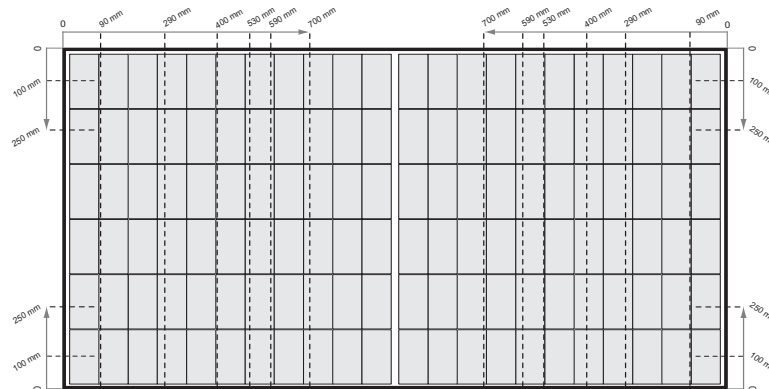
Afb. 3-3 Klemmen van de panelen van de serie REC Alpha Pure 2 met korte rails
