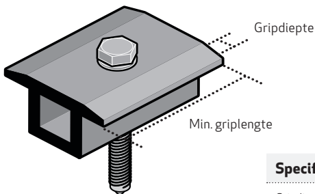
Afb. 1 Specificaties klemmen
