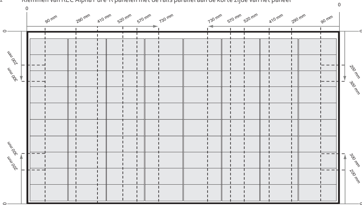
Afb. 4-1 Klemmen van REC Alpha Pure-R panelen met de rails parallel aan de korte zijde van het paneel
