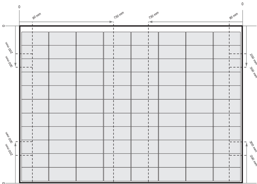
Afb. 5-2 Klemmen van REC Alpha Pure-RX panelen met de rails parallel aan de lange zijde van het paneel
