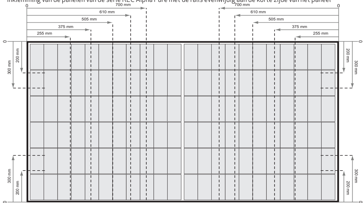
Afb. 2-1 Inklemming van de panelen van de serie REC Alpha Pure met de rails evenwijdig aan de korte zijde van het paneel
