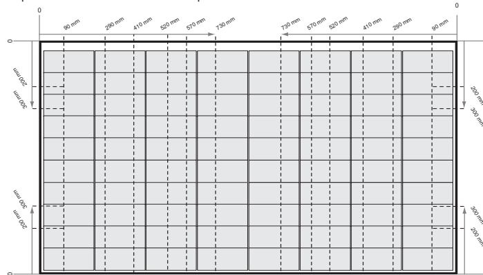
Afb. 4-3 Klemmen van de panelen van de serie REC Alpha Pure-R met korte rails
