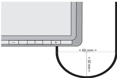
Afb. 6 Minimale dkabelafstand
