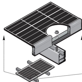
Afb. 4 Montage gaten installatie voorbeeld
