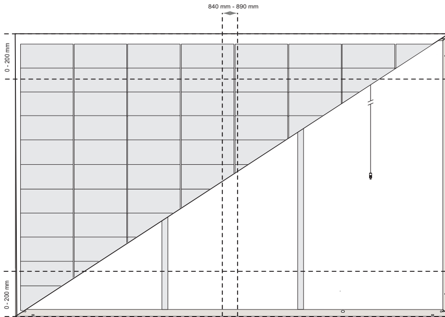
Afb. 5-5 Gemengde zespuntsmontage van panelen uit de REC Alpha Pure-RX-serie met korte rails
