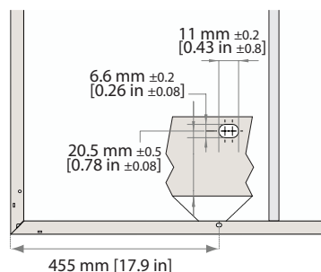
Afb. 3 Montagegaten: REC Alpha panelen
