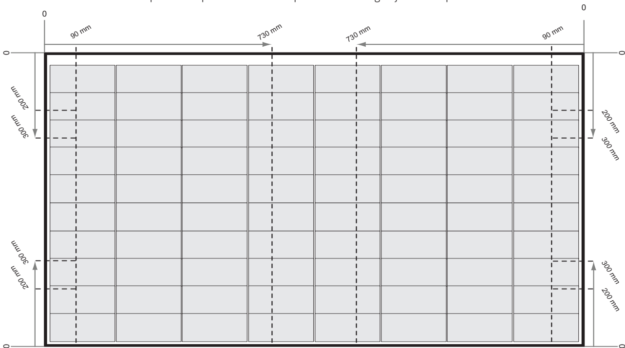
Afb. 4-2 Klemmen van REC Alpha Pure-R panelen met de rails parallel aan de lange zijde van het paneel
