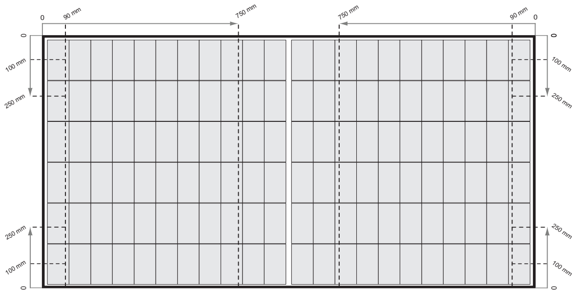
Afb. 3-2 Klemmen van REC Alpha Pure 2 serie panelen met Rails parallel aan de lange zijde van het paneel
