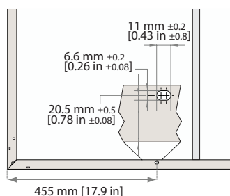
fig. 3 Trous de montage : Panneaux REC Alpha
