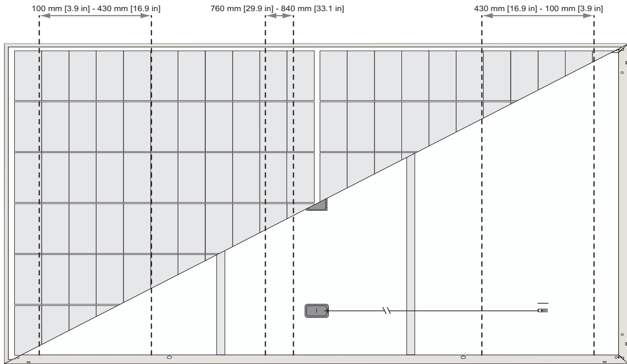
fig. 2-4 Zones de serrage de la configuration de montage à six points : Série REC Alpha Pure
