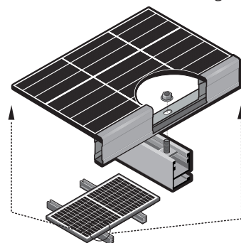
fig. 4 Exemple d'installation des trous de montage
