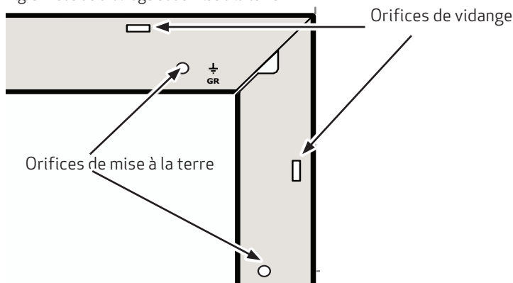
fig. 5 Trous de drainage et de mise à la terre
