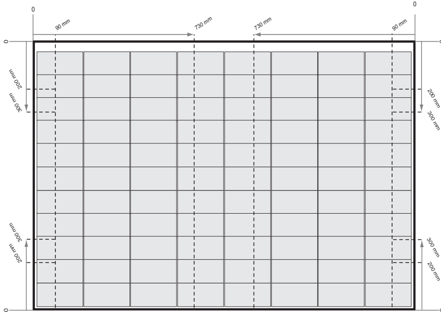
fig. 5-2 Fixation des panneaux de la série REC Alpha Pure-RX avec les rails parallèles au côté long du panneau
