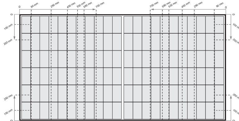
fig. 3-3 Fixation des panneaux de la série REC Alpha Pure 2 à l'aide de rails courts
