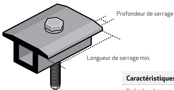
fig. 1 Spécifications des colliers de serrage
