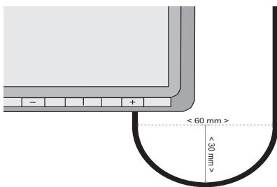
fig. 6 d Distance minimale du câble
