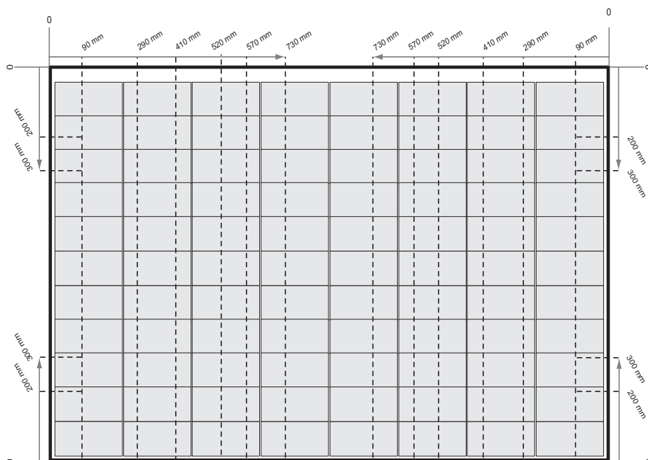
fig. 5-1 Fixation des panneaux de la série REC Alpha Pure-RX avec les rails parallèles au côté court du panneau
