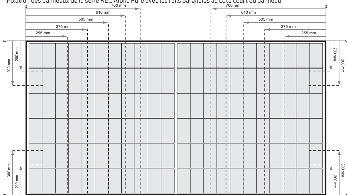
fig. 2-1 Fixation des panneaux de la série REC Alpha Pure avec les rails parallèles au côté court du panneau
