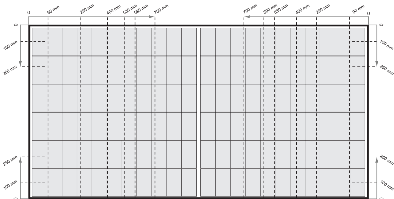
fig. 3-1 Fixation des panneaux de la série REC Alpha Pure 2 avec les rails parallèles au côté court du panneau
