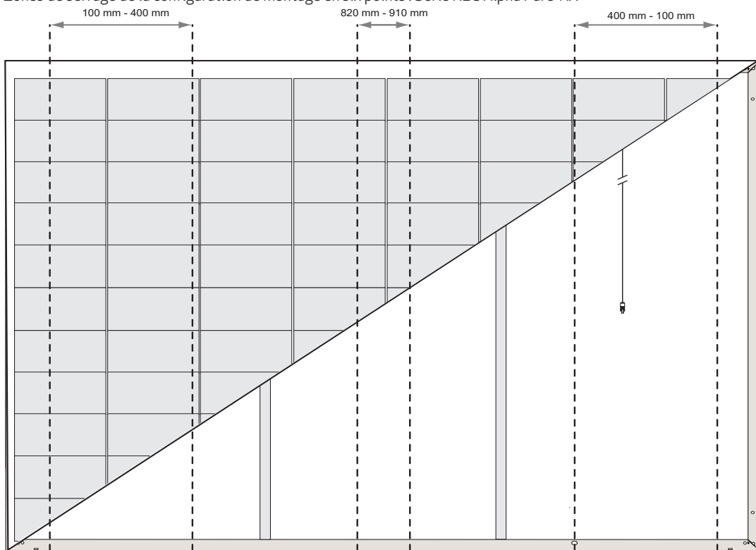
fig. 5-4 Zones de serrage de la configuration de montage en six points : Série REC Alpha Pure-RX
