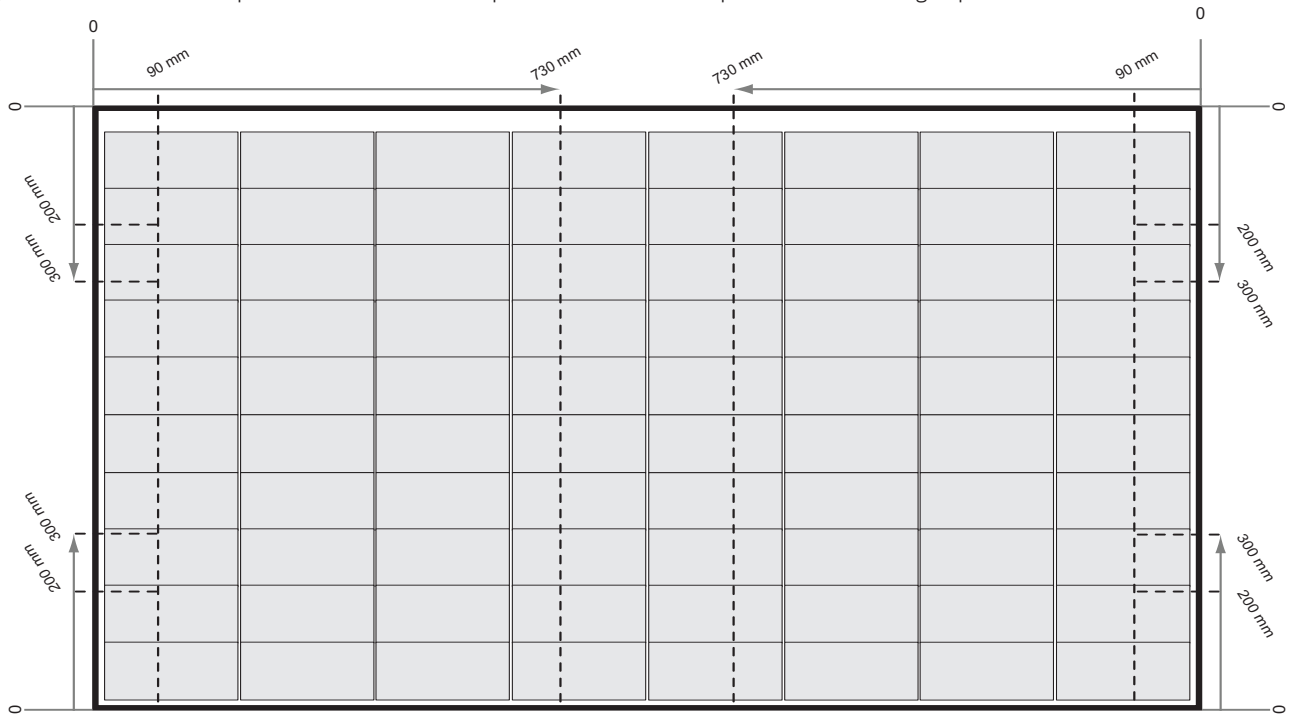
fig. 4-2 Fixation des panneaux de la série REC Alpha Pure-R avec les rails parallèles au côté long du panneau
