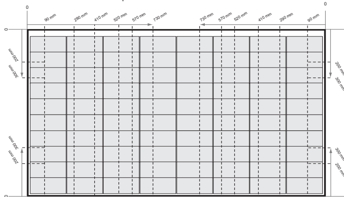
fig. 4-3 Fixation des panneaux de la série REC Alpha Pure-R à l'aide de rails courts
