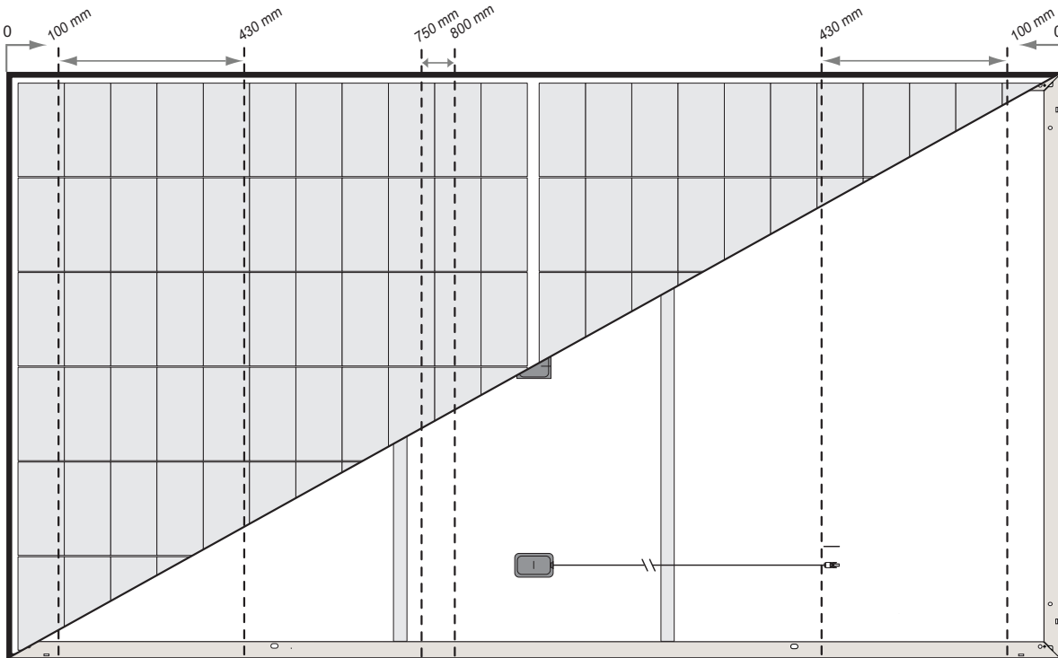
fig. 3-4 Zones de serrage de la configuration de montage en six points : Série REC Alpha Pure 2
