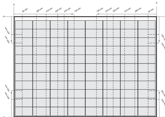
fig. 5-3 Fixation des panneaux de la série REC Alpha Pure-RX à l'aide de rails courts
