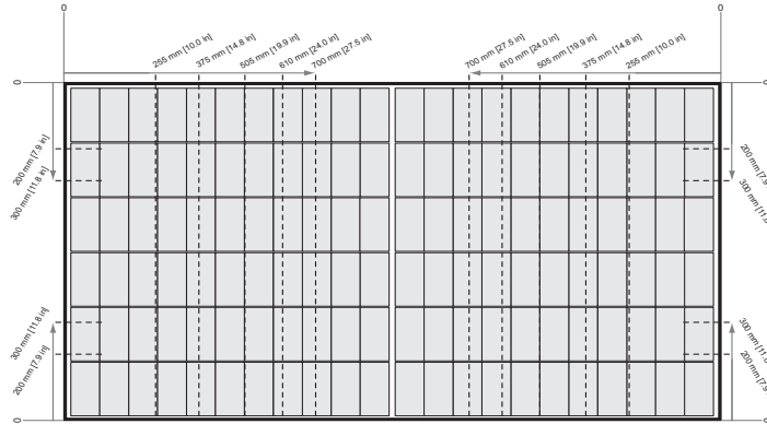
fig. 2-3 Fixation des panneaux de la série REC Alpha Pure à l'aide de rails courts
