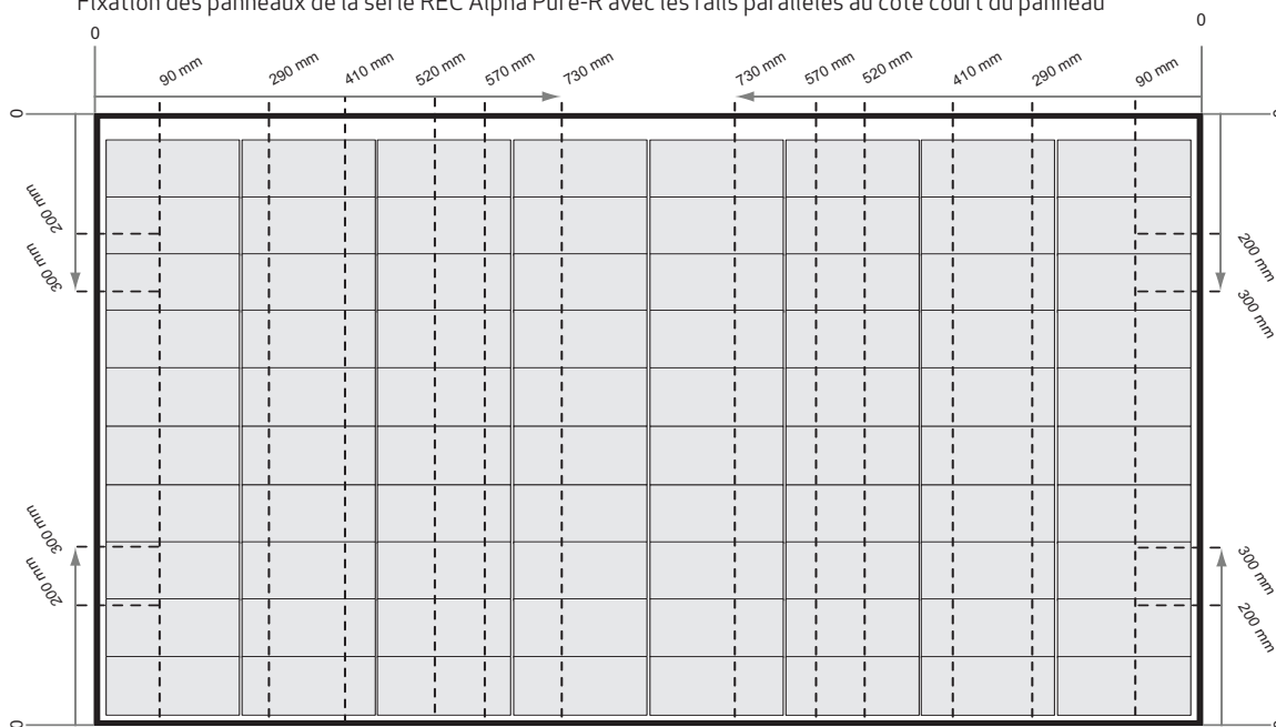
fig. 4-1 Fixation des panneaux de la série REC Alpha Pure-R avec les rails parallèles au côté court du panneau
